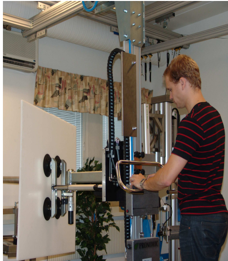
Hantering av skivmaterial med vakuum.
